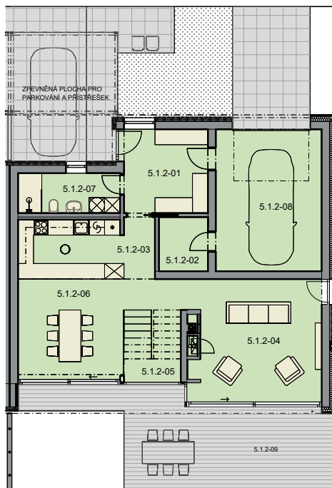
PŮDORYS 1NP 1:150
