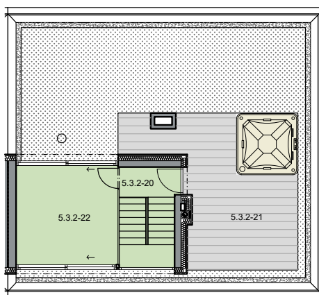
PŮDORYS 3NP 1:150
